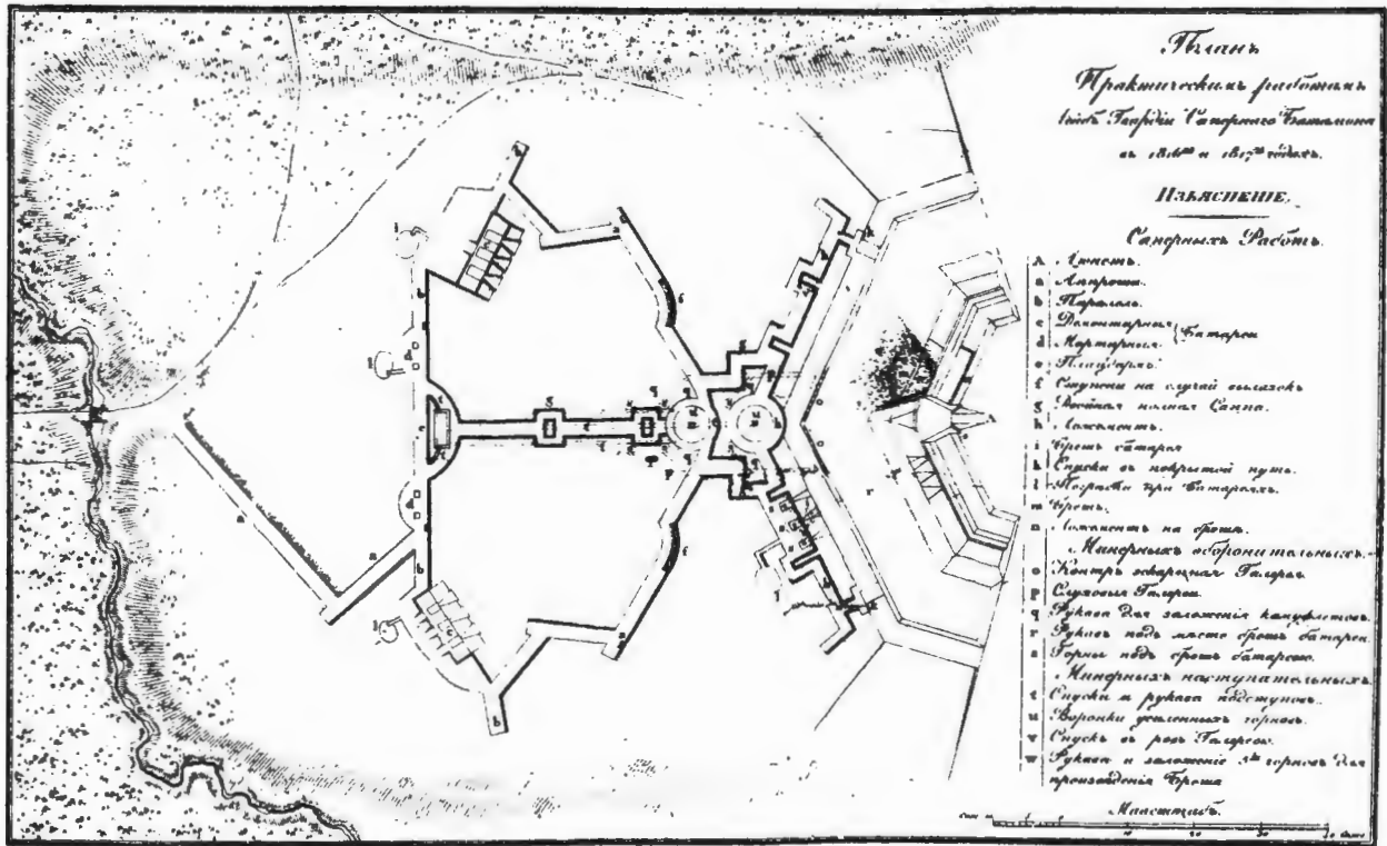
Типы сапныхъ работъ.
