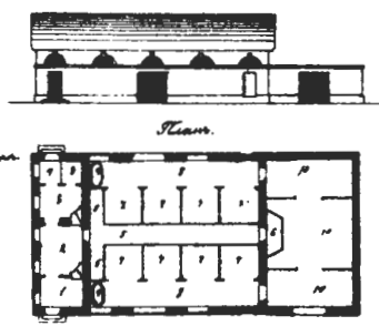
План фасады и проходы конюшни завода Гренадерского полка в Штабе Гренадерского полка Архангела Гавриила
