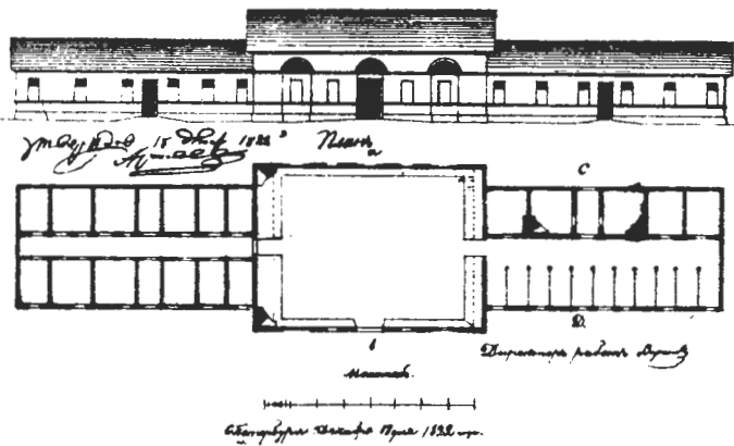
План и фасад конюшен завода в Штабе Гренадерского Полка Архангела Гавриила
