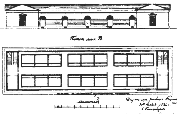
План фасады и проходы конюшни завода Гренадерского полка в Штабе Гренадерского полка Архангела Гавриила
