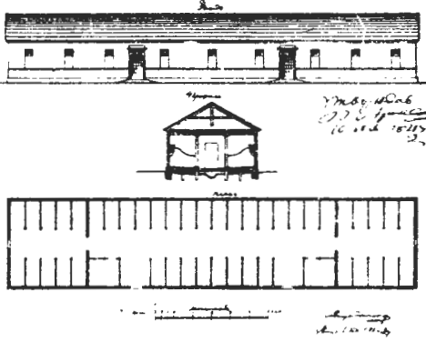
План фасады и проходы конюшни завода Гренадерского полка в Штабе Гренадерского полка Архангела Гавриила
