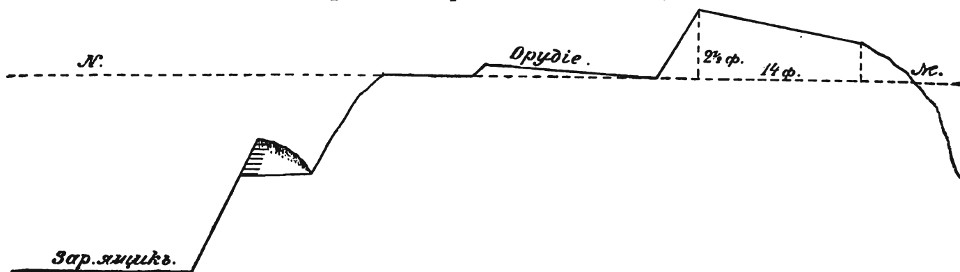
Профиль батареи № 1. По линіи М.
