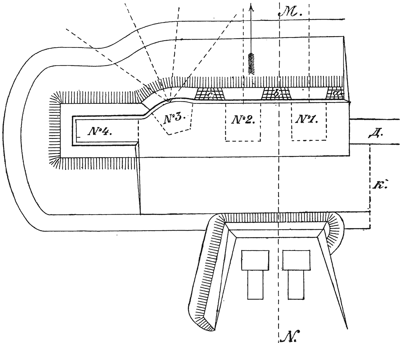
Планъ батареи № 1.
